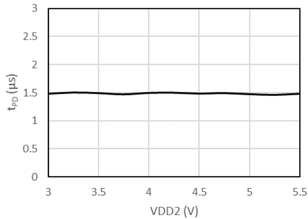
图 7-21 输入输出信号延时 vs VDD2
