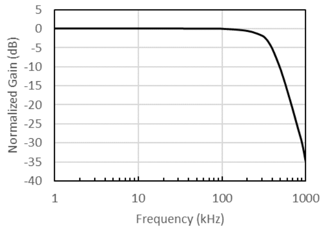
图 7-24 归一化增益 vs 频率
