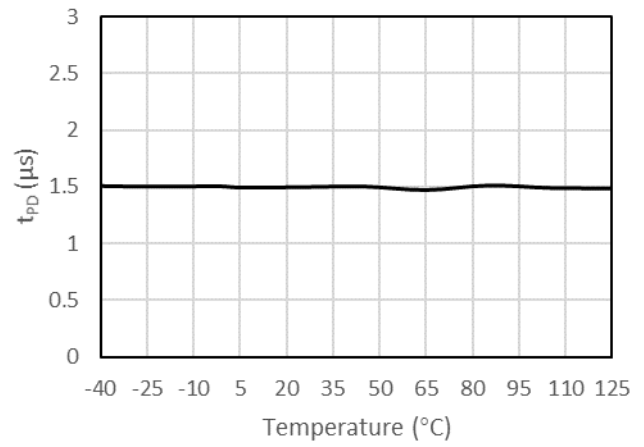
图 7-20 输入输出信号延时 vs 温度
