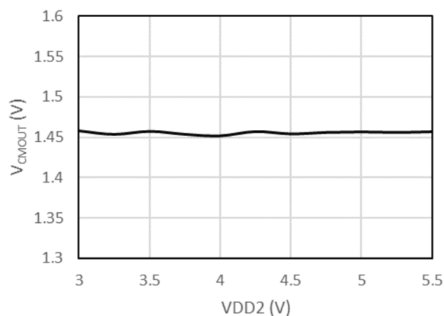
图 7-17 低边共模输出电压 vs VDD2
