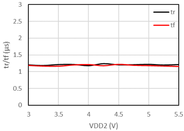
图 7-19 输出上升下降时间 vs VDD2
