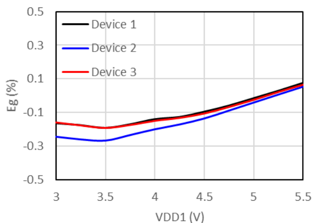
图 7-2 增益误差 vs VDD1
