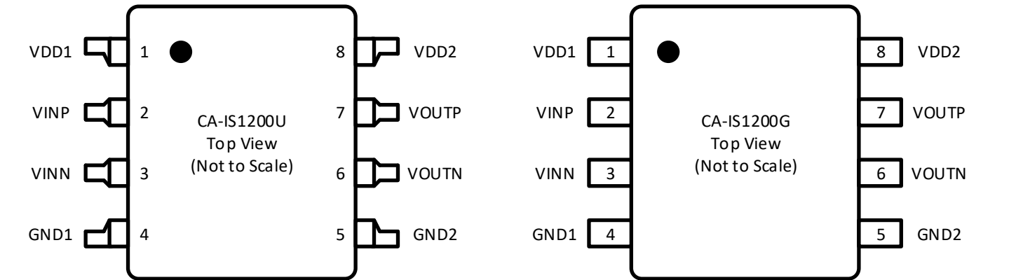
图 6-1 CA-IS1200 引脚配置
