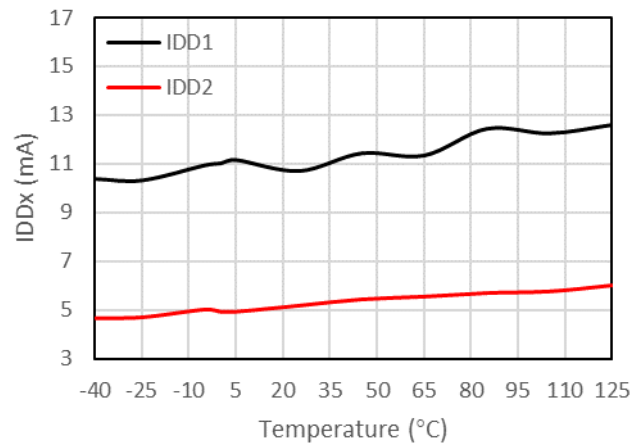
图 7-22 供电电流 vs 温度
