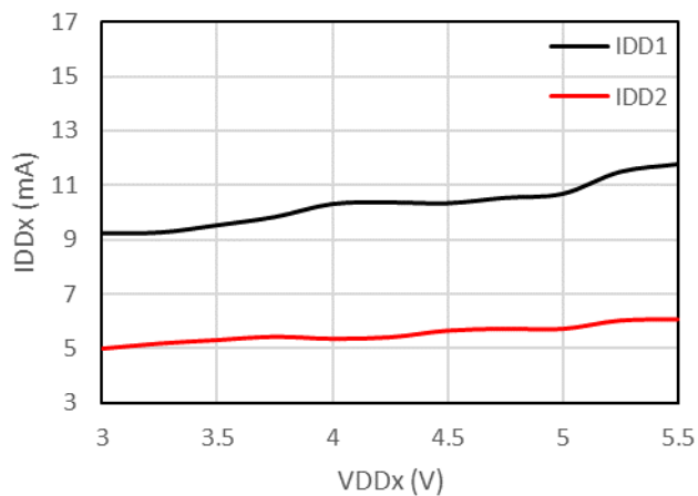
图 7-23 供电电流 vs 供电电压
