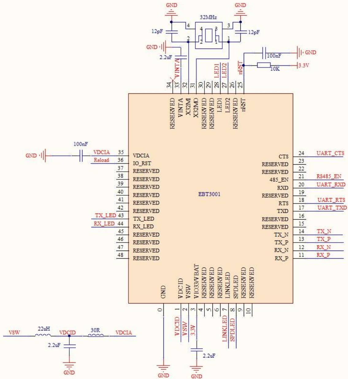
EBT3001最小系统参考电路
