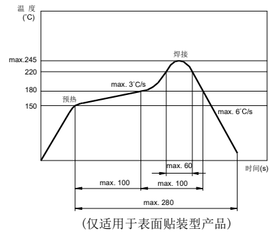
回流焊, PCB板面温度(推荐焊接温度)
