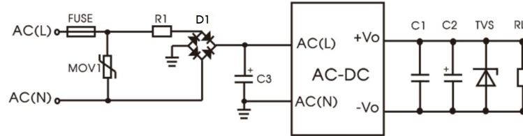
图 3: EMC 更高要求推荐电路
