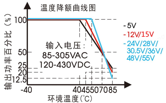
有铝板散热
