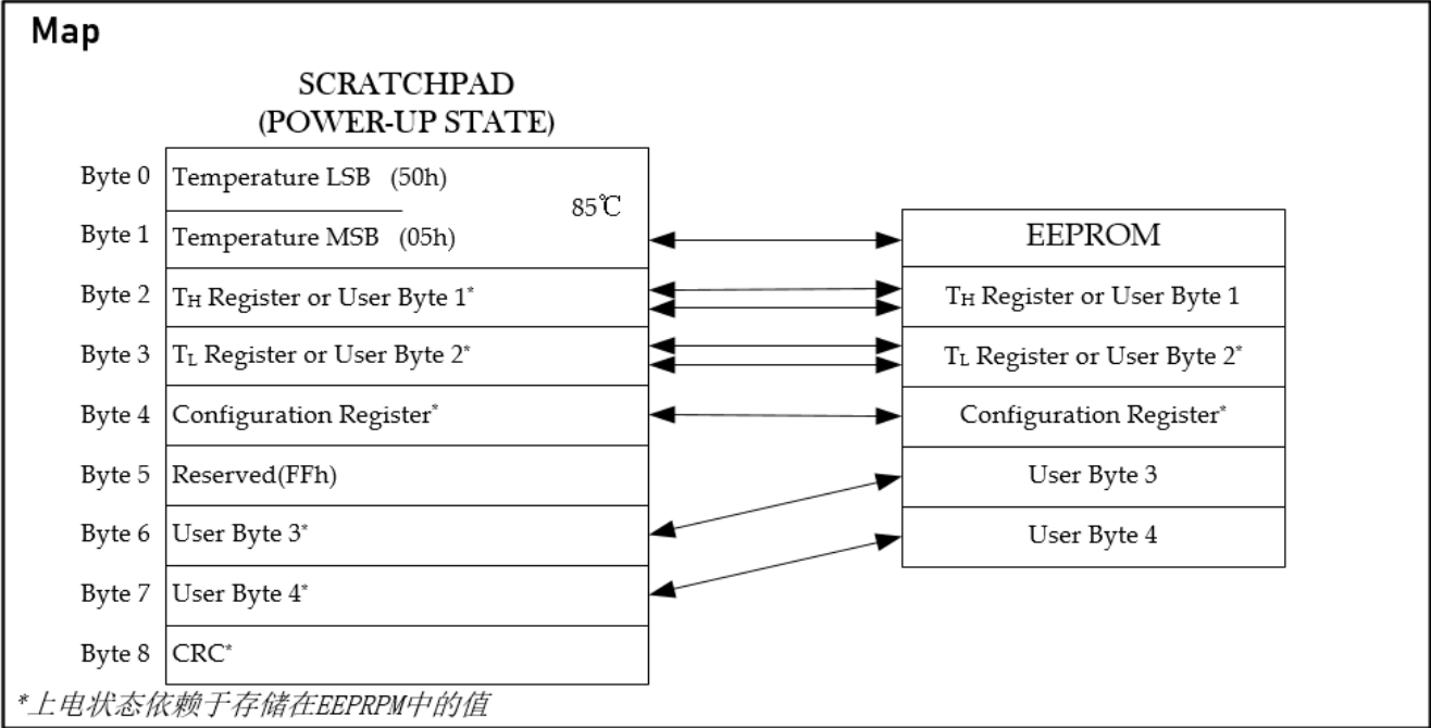
图 7. MDS18B20存储器图
