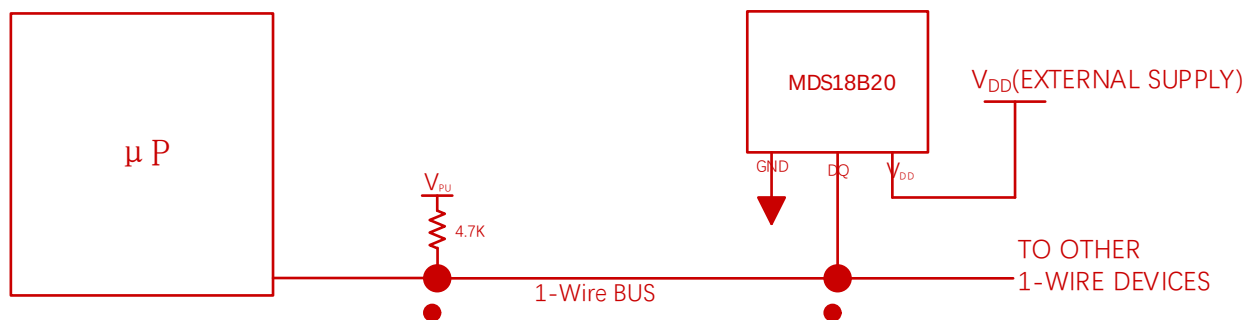
图 5. 使用外部电源为 MDS18B20供电
