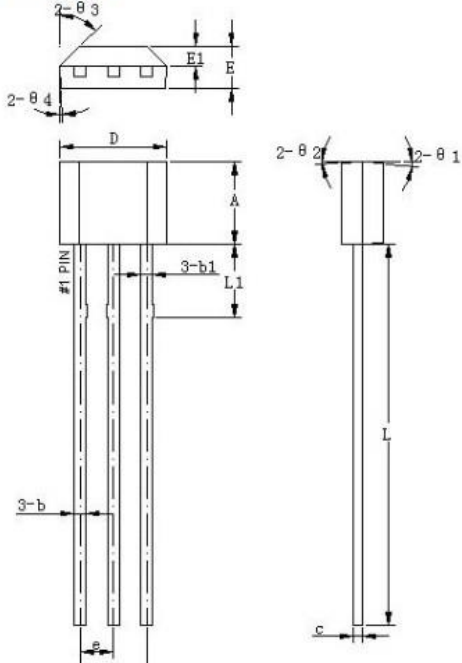
TO-92S-A1
