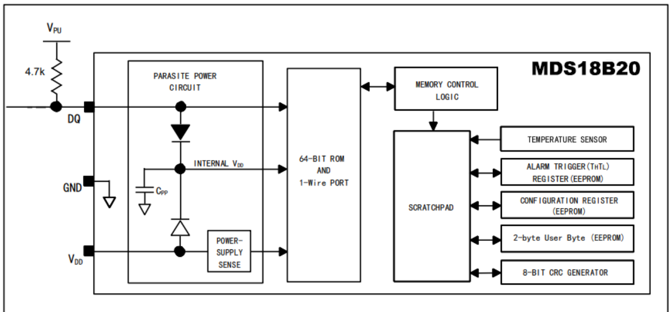
图 1. MDS18B20结构框图
