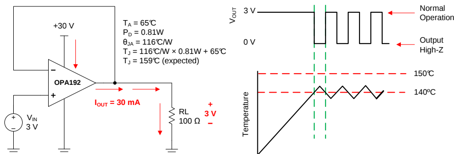
图 59. 过热保护
