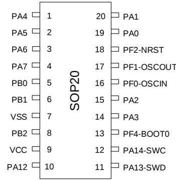
图 3-7 SOP20 Pinout1 PY32F003F1xS
