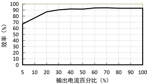
URB2405LD-40W(H)R3 效率Vs输出负载 ( V_{\text{in}}=24\text{V} )
