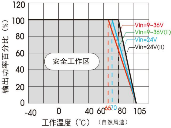
URB2412LD-40W(H)R3 温度降额曲线图
