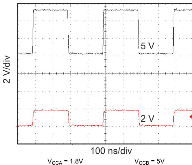
图 9-2. 2.5MHz 信号的电平转换
